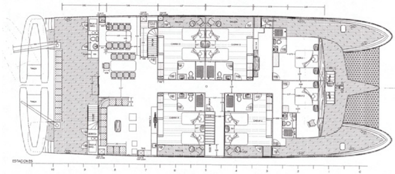
CUBIERTA PRINCIPAL MAIN DECK
