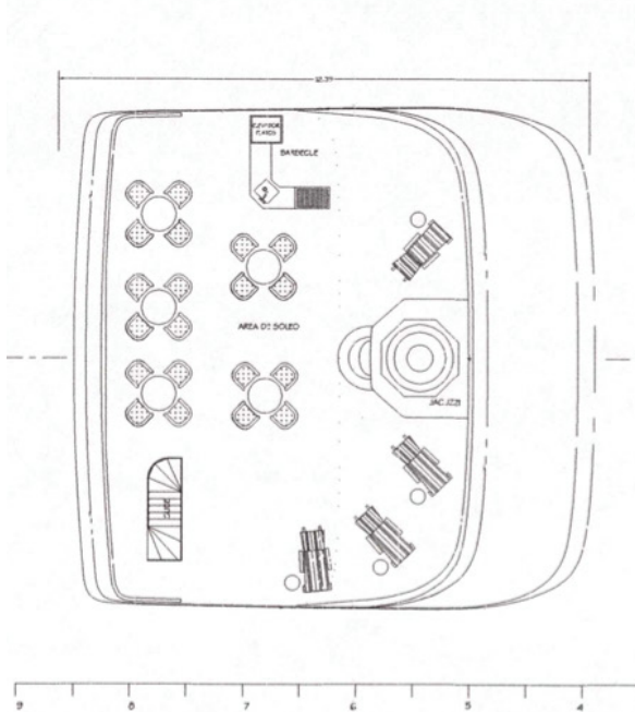
CUBIERTA DE SOL SUN DECK
