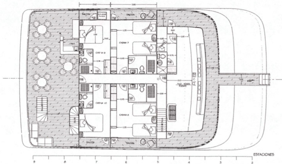
CUBIERTA SUPERIOR UPPER DECK
